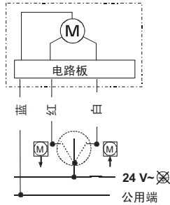
增量控制型号接线图
