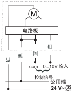
比例控制型号接线图
